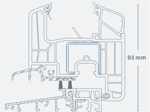
Nouveau: seuil de porte-balcon sans obstacle Plan: 1:2
